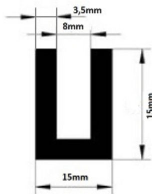
USZCZELKA W57
